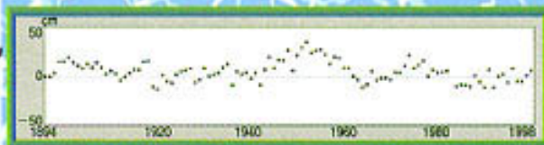
HOSOJIMA / 年平均潮位の変化
