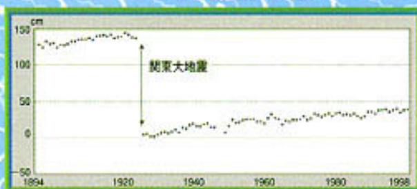
ABURATSUBO / 年平均潮位の変化
